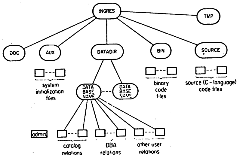
Fig. 3. The INGRES subtree
