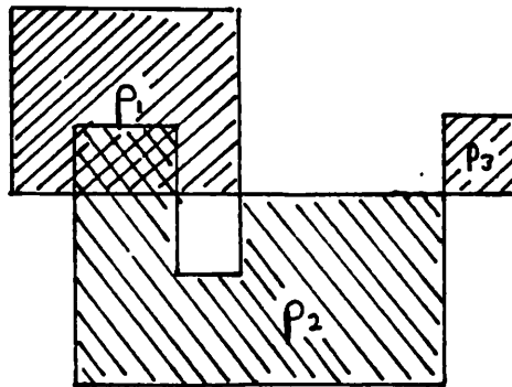
Fig. 2.2: p_1 + p_2 + p_3
