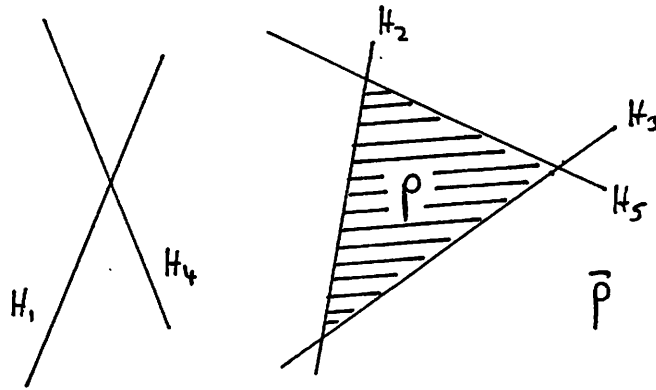
Fig. 4.1: \mathbf{h}_p = (0, 1, -1, 0, -1) , x_{\bar{p}} = -1 \cdot H_2 + 1 \cdot H_3 + 1 \cdot H_5
