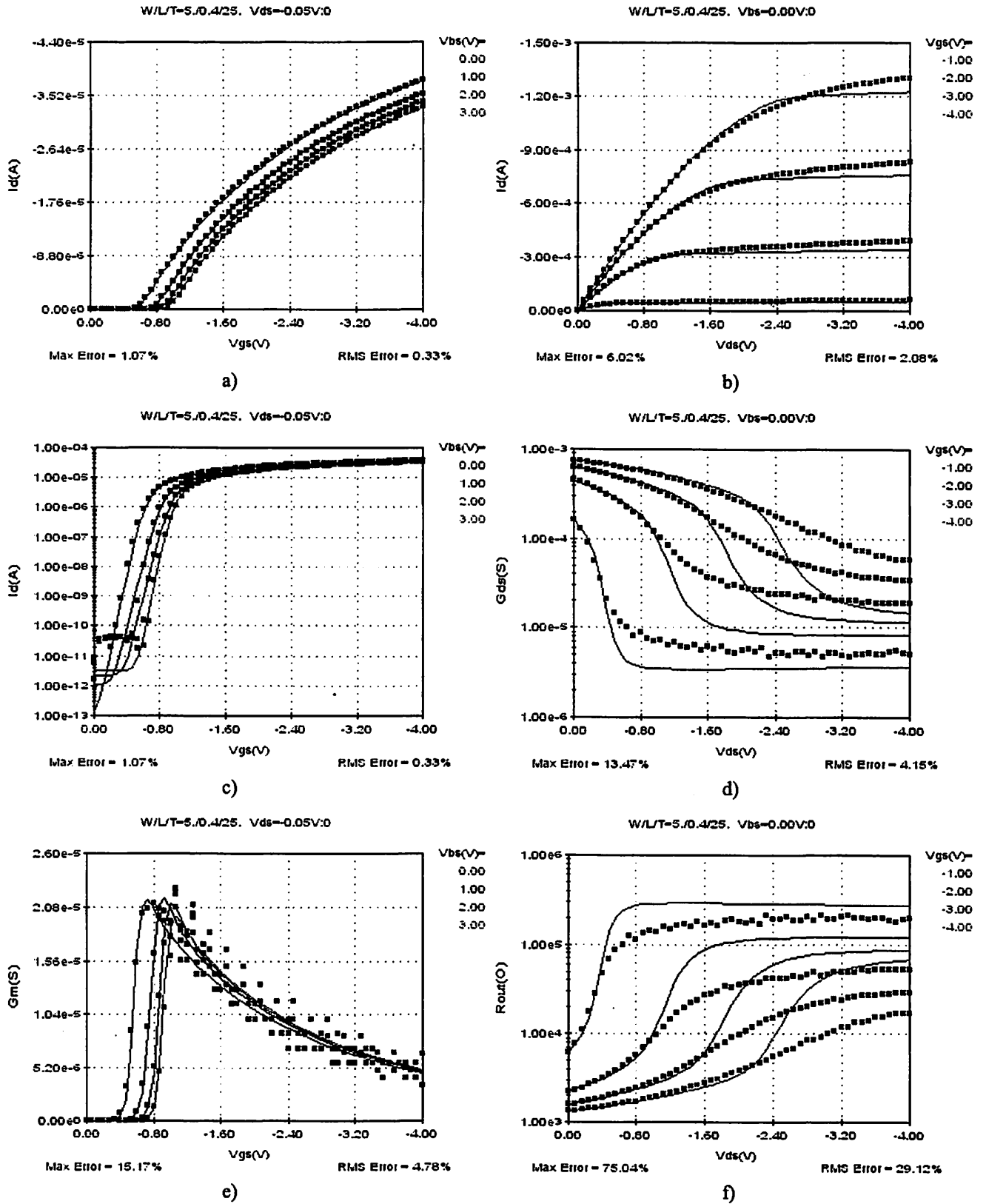
Fig 33 - L=0.4\mu m W=5\mu m PMOS
