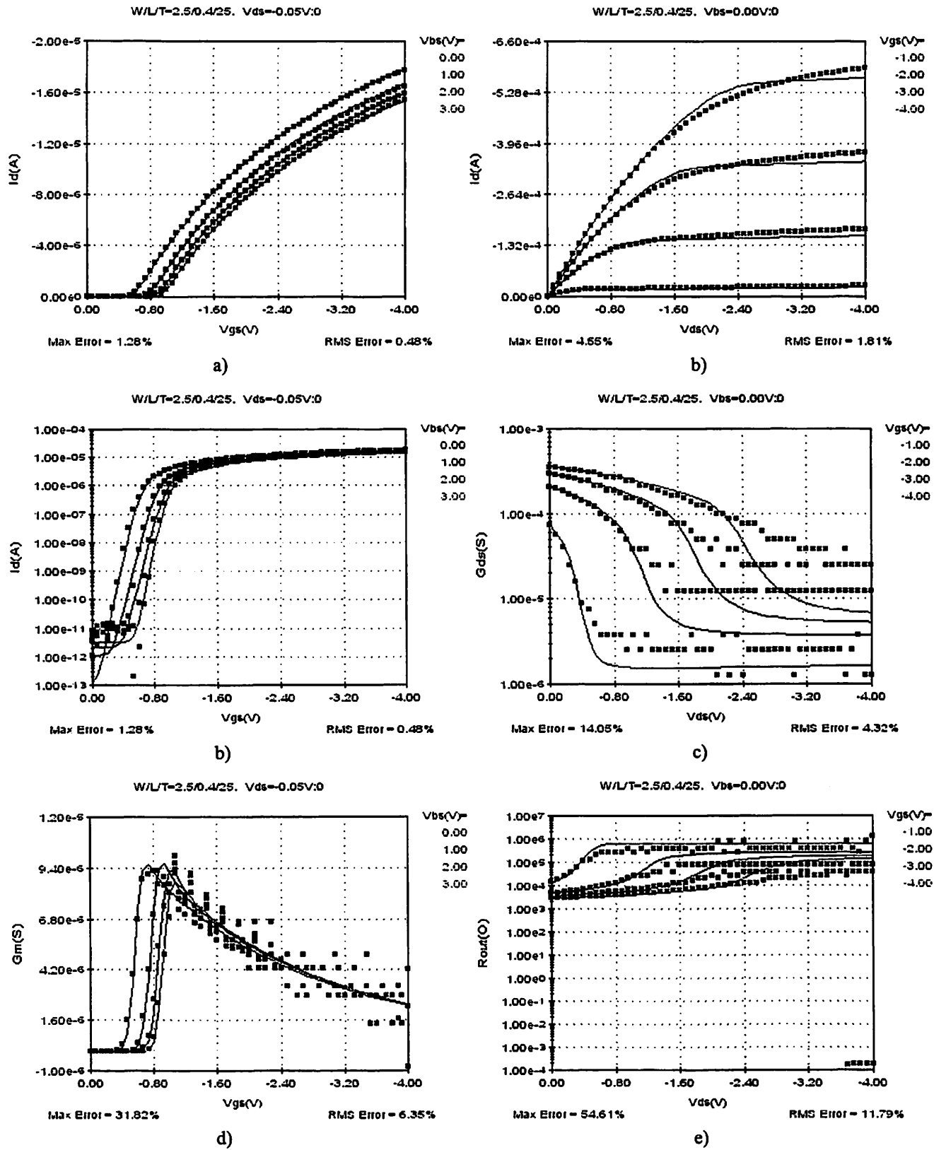
Fig 32 - L=0.4um W=2.5um PMOS
