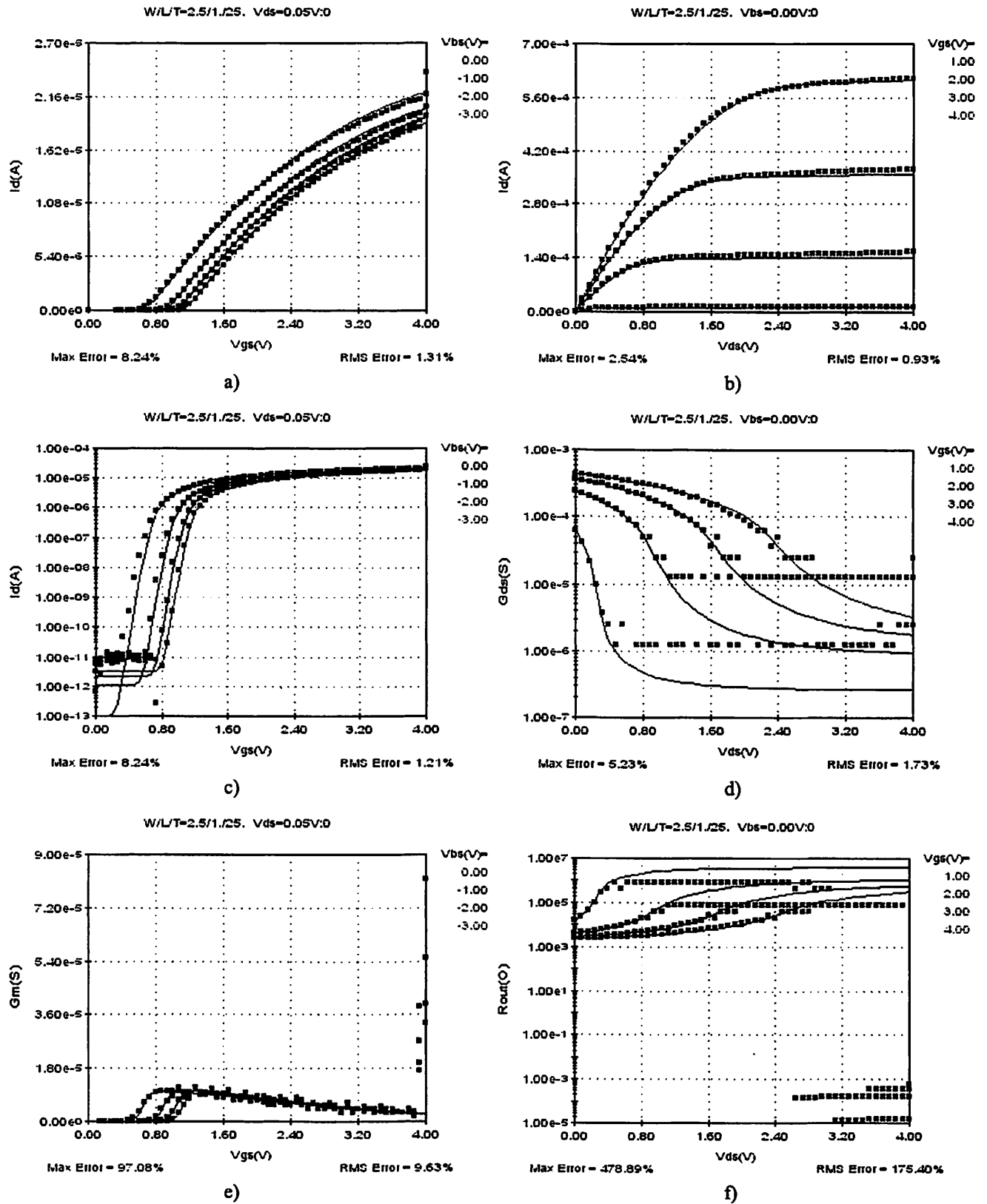
Fig 31 - L=1um W=2.5um NMOS
